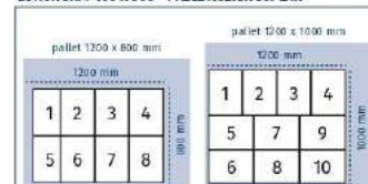
EURONORM 400 X 300 - PALLETISERINGSPLAN
